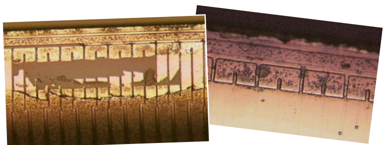
Beispiele eines durch ein minderwertiges Farbband zerstörten Druckkopfes
